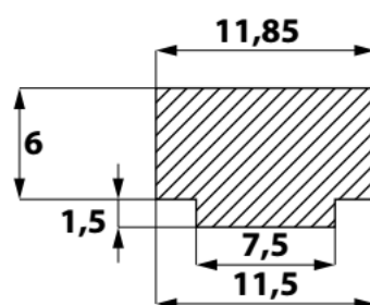
PRZEKRÓJ A - A
